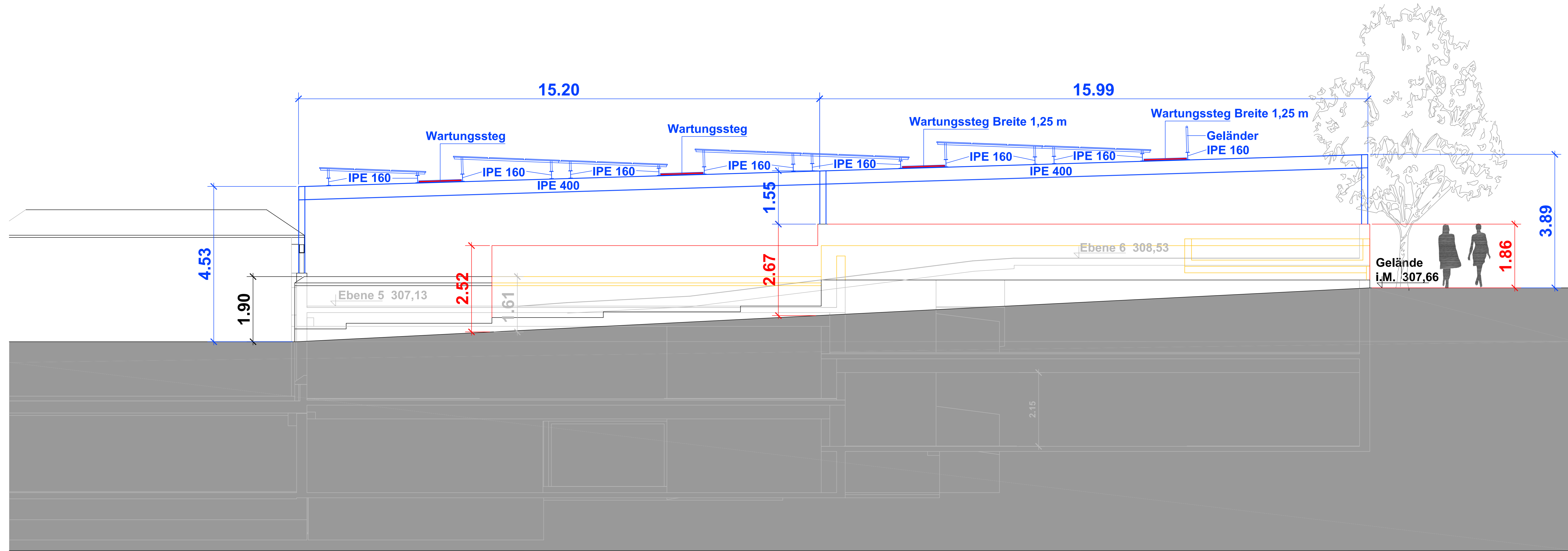
Westansicht Eugenstraße PV-Anlage auf Stahlkonstruktion mit Wartungsstegen
