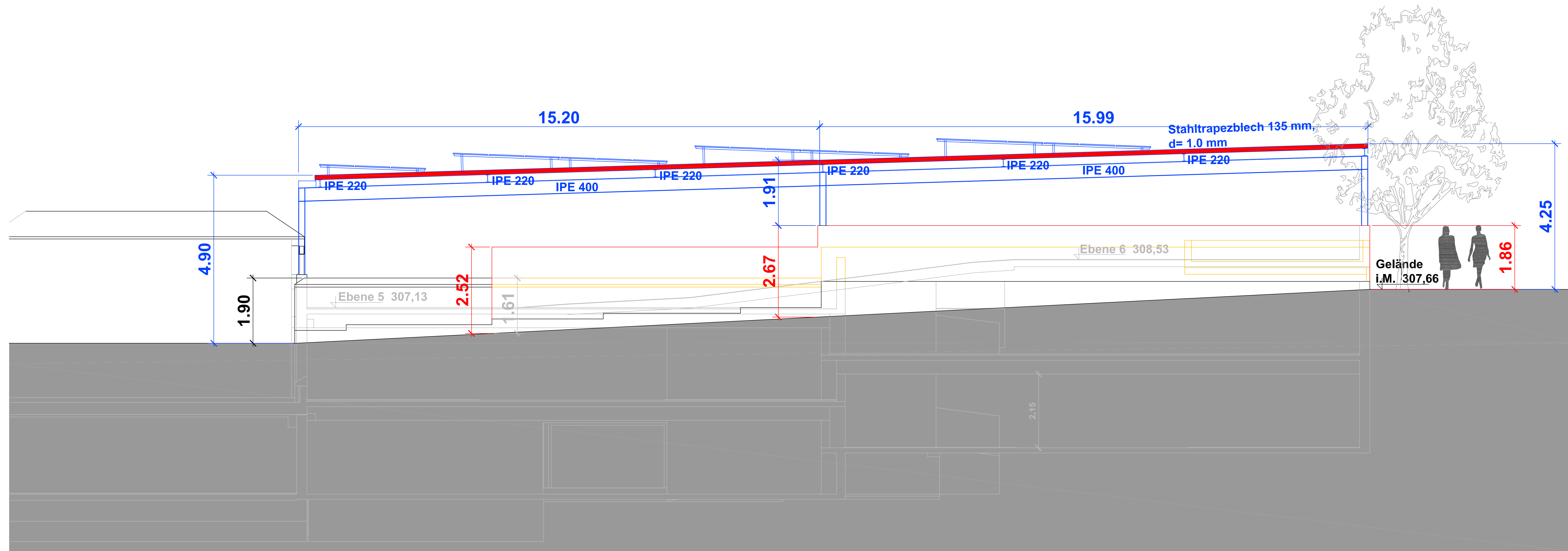
Westansicht Eugenstraße PV-Anlage auf geschlossener Dachdeckung
